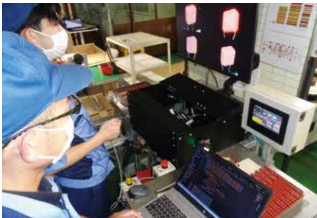
外観検査の画像処理化による製品検査
